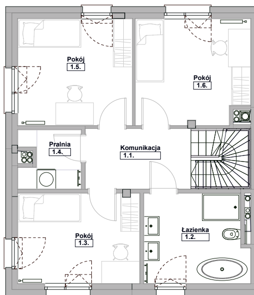
Rzut piętra
