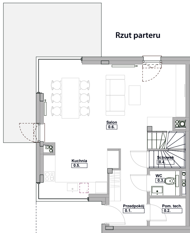
Rzut parteru
