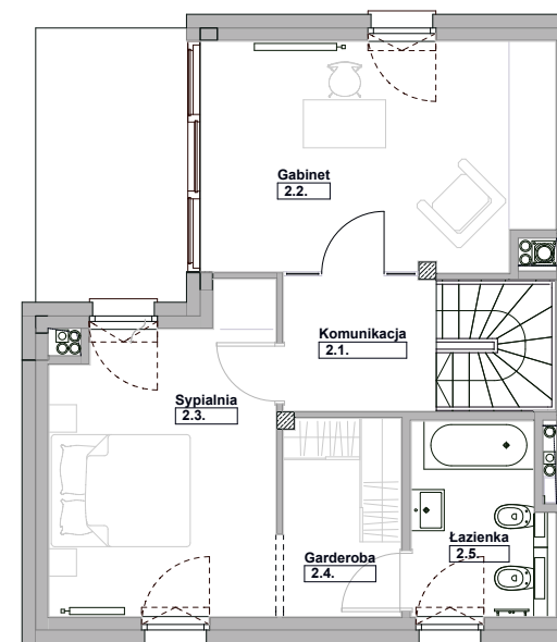
Rzut 2 piętra
